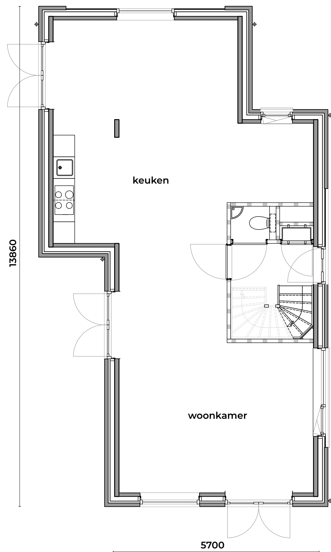
Begane grond
