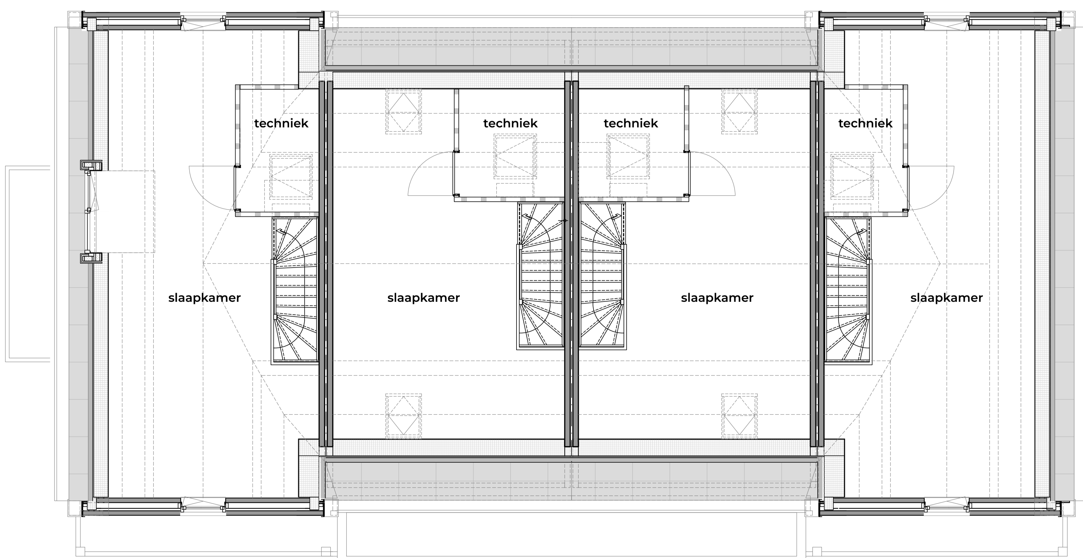
Tweede verdieping
