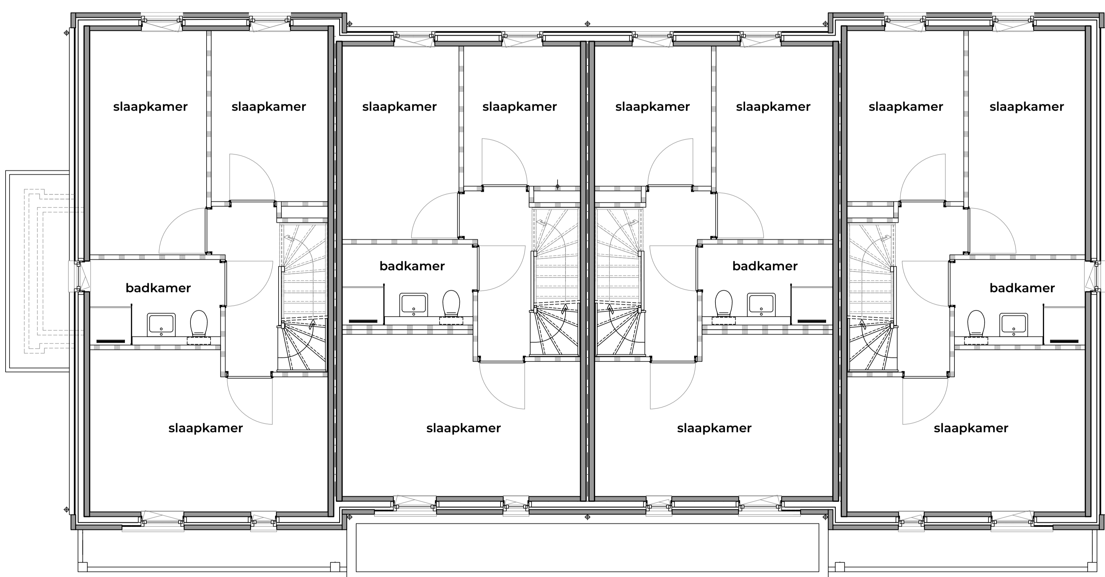
Eerste verdieping
