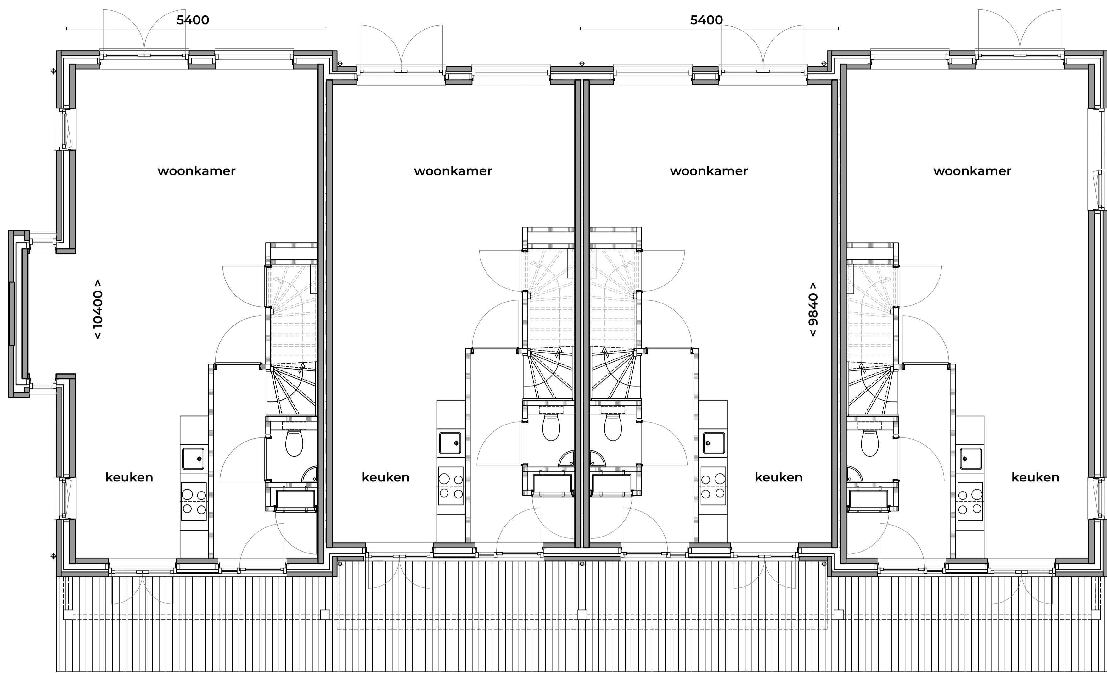
Begane grond
